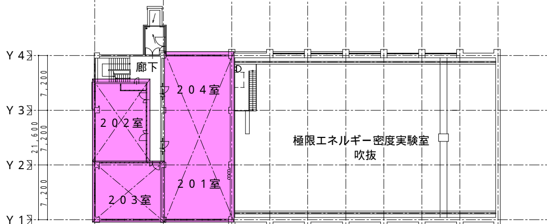
極限センター2号棟 2階平面図
